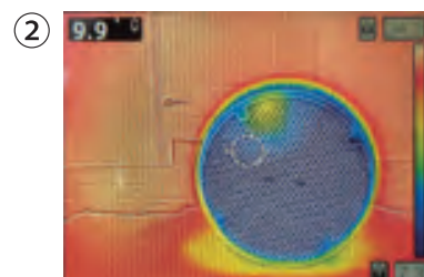
室内に70秒間給気した後のセラミックの状態。熱がセラミックから放熱されていきます。
