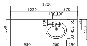
■鳥瞰図
