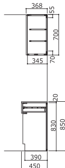
■断面図(右)
