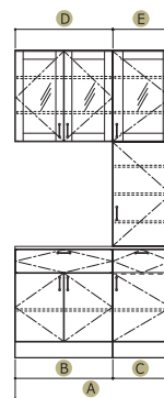
■正面図
