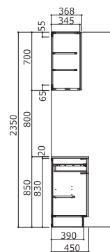
■断面図(左)
