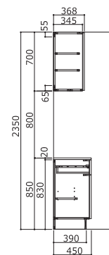
■断面図(左)
