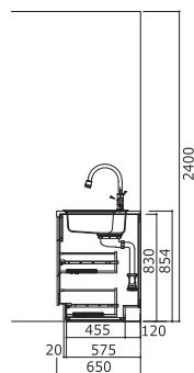
■断面図(シンク側)
