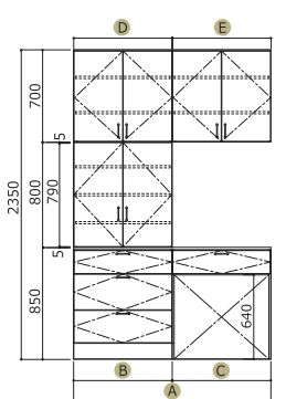
■正面図
