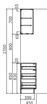
■断面図(左)
