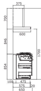
■断面図(加熱機器側)
