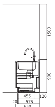
■断面図(シンク側)
