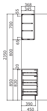
■断面図(左)
