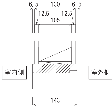
上枠納まり
