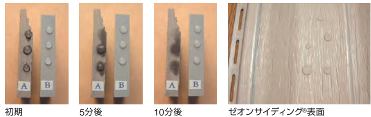
外装材への水滴滴下試験（窯業系サイディングAとゼオンサイディング®B）
