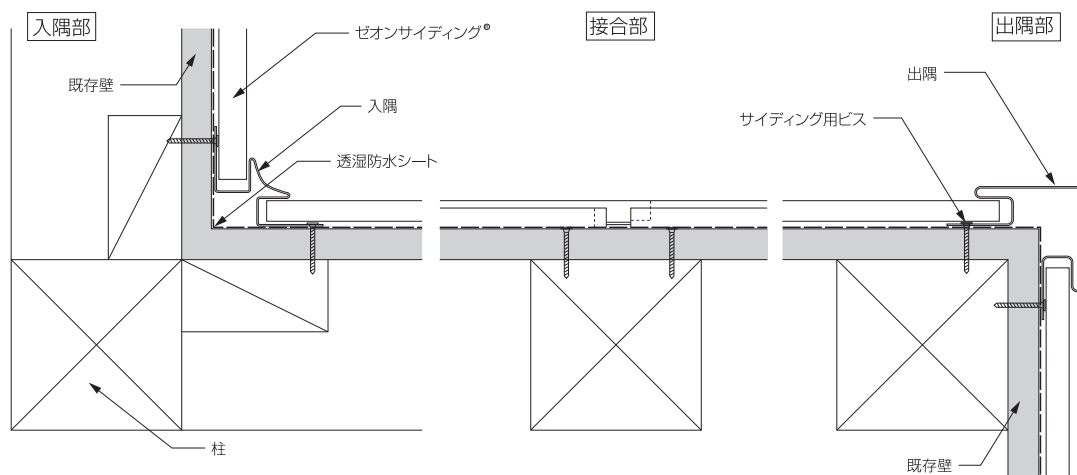
入隅部・ジョイント部・出隅部納まり図(横断面図)
