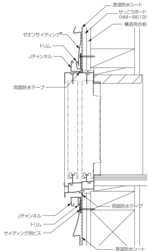
窓回り納まり図(断面図)
