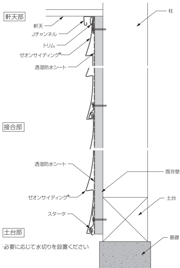
基本納まり図(断面図) ※胴縁を使わない例
