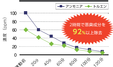
アンモニア、トルエンの除去実験
