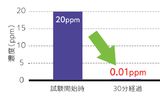
硫化水素の除去実験
