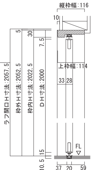
上下レール
