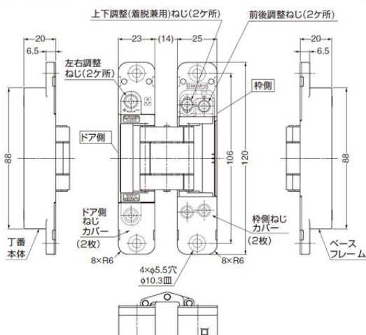
a. 分解図
