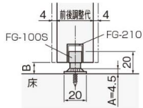
下部ガイド
