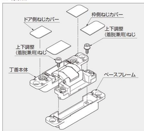
b. ドア取付方法
