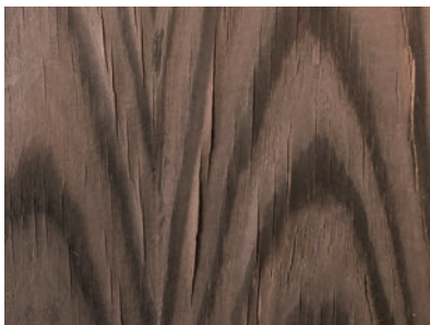
塗料の拭き取り不足による表面割れ
